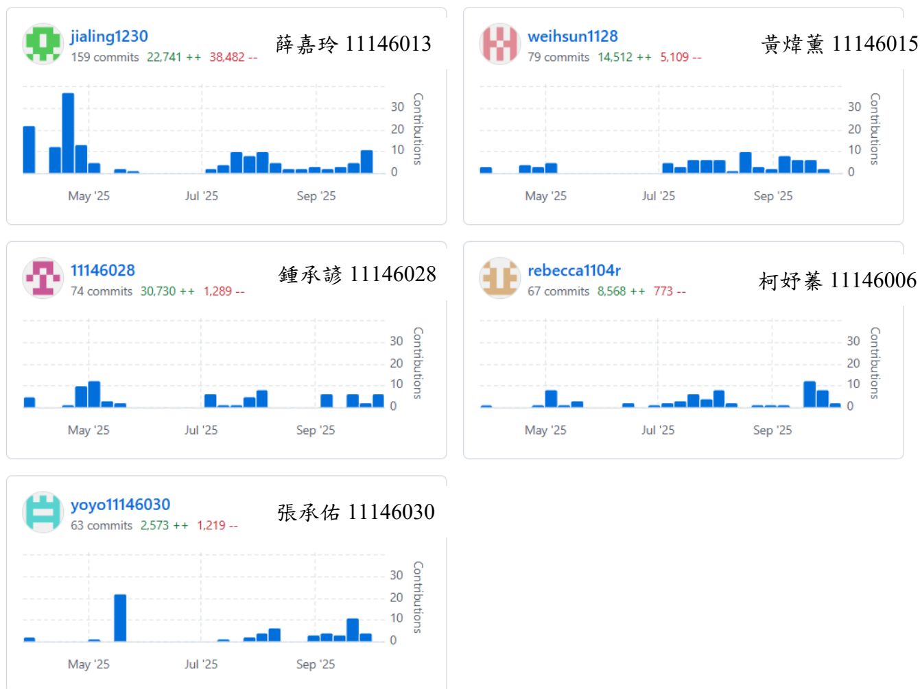
圖 4-3-1 Github 頁面
