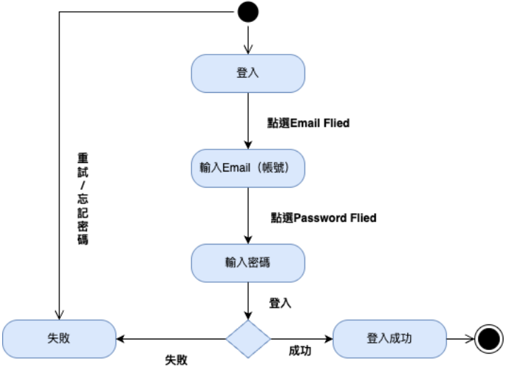
圖 7-4-2 狀態圖-登入
