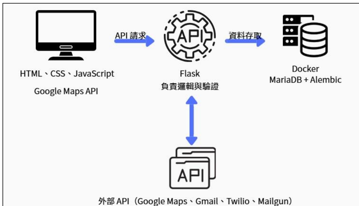
圖 3-1-1 系統架構圖
