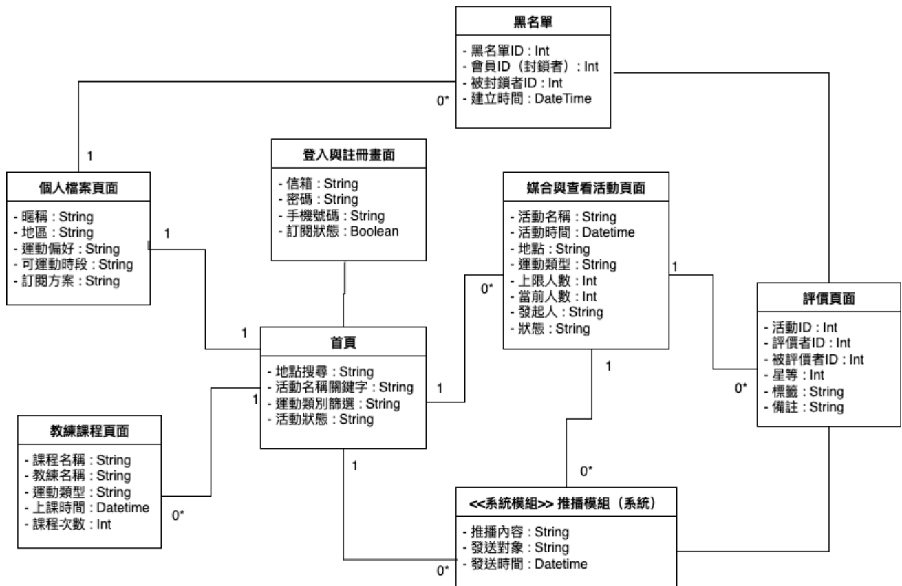
圖 5-4-1 分析類別圖
