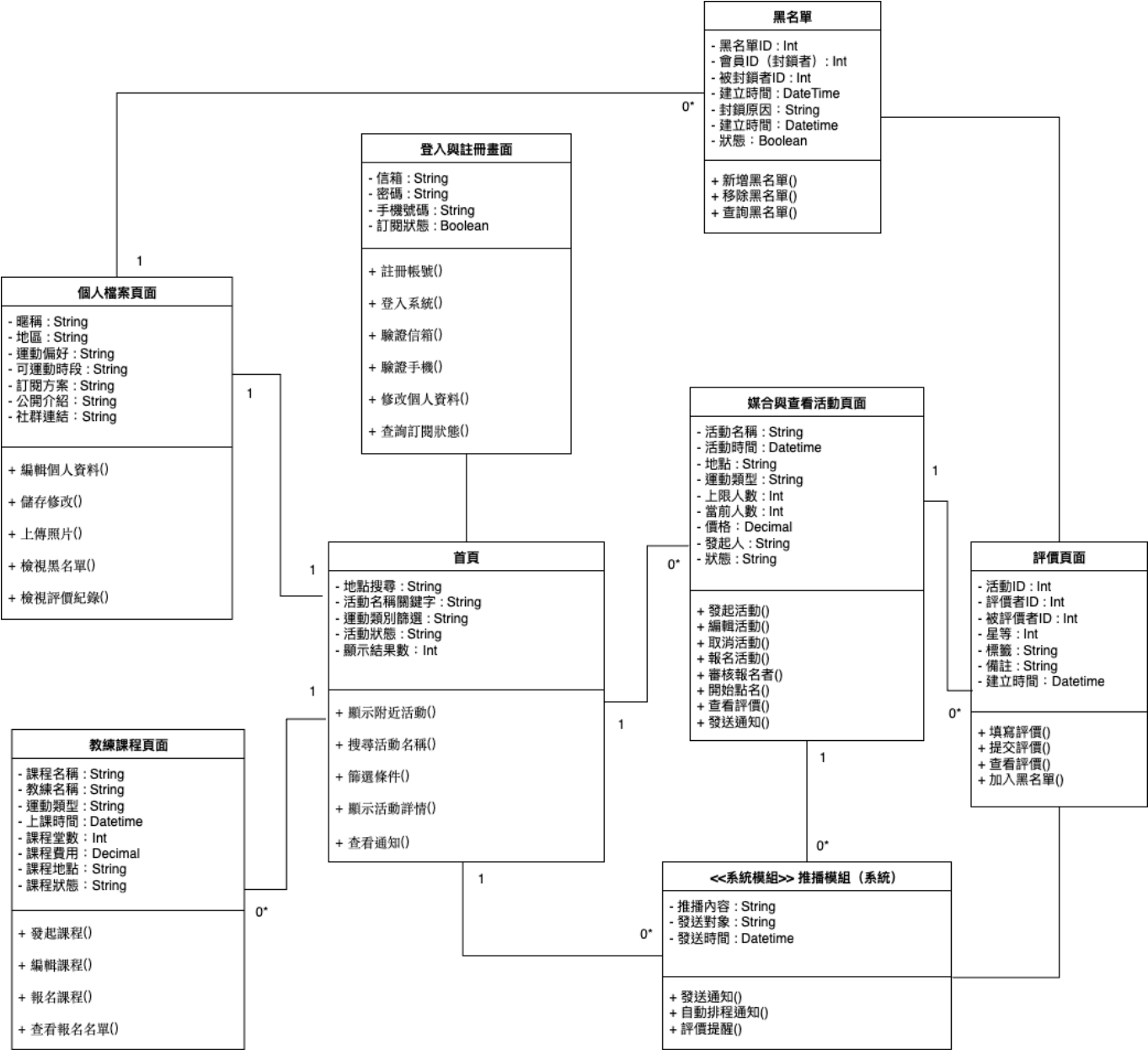
圖 6-2-1 設計類別圖
