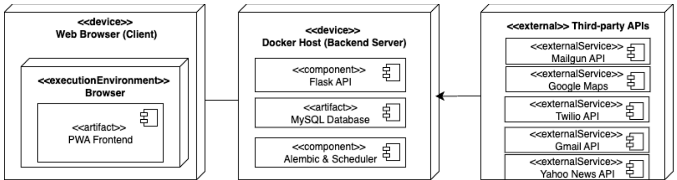
圖 7-1-1 佈署圖
