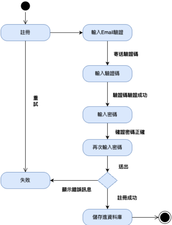
圖 7-4-1 狀態圖-註冊
