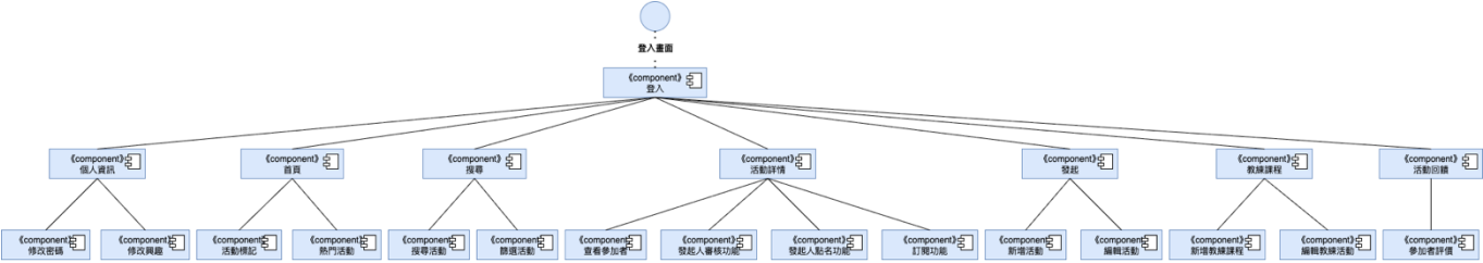
圖 7-3-1 元件圖
