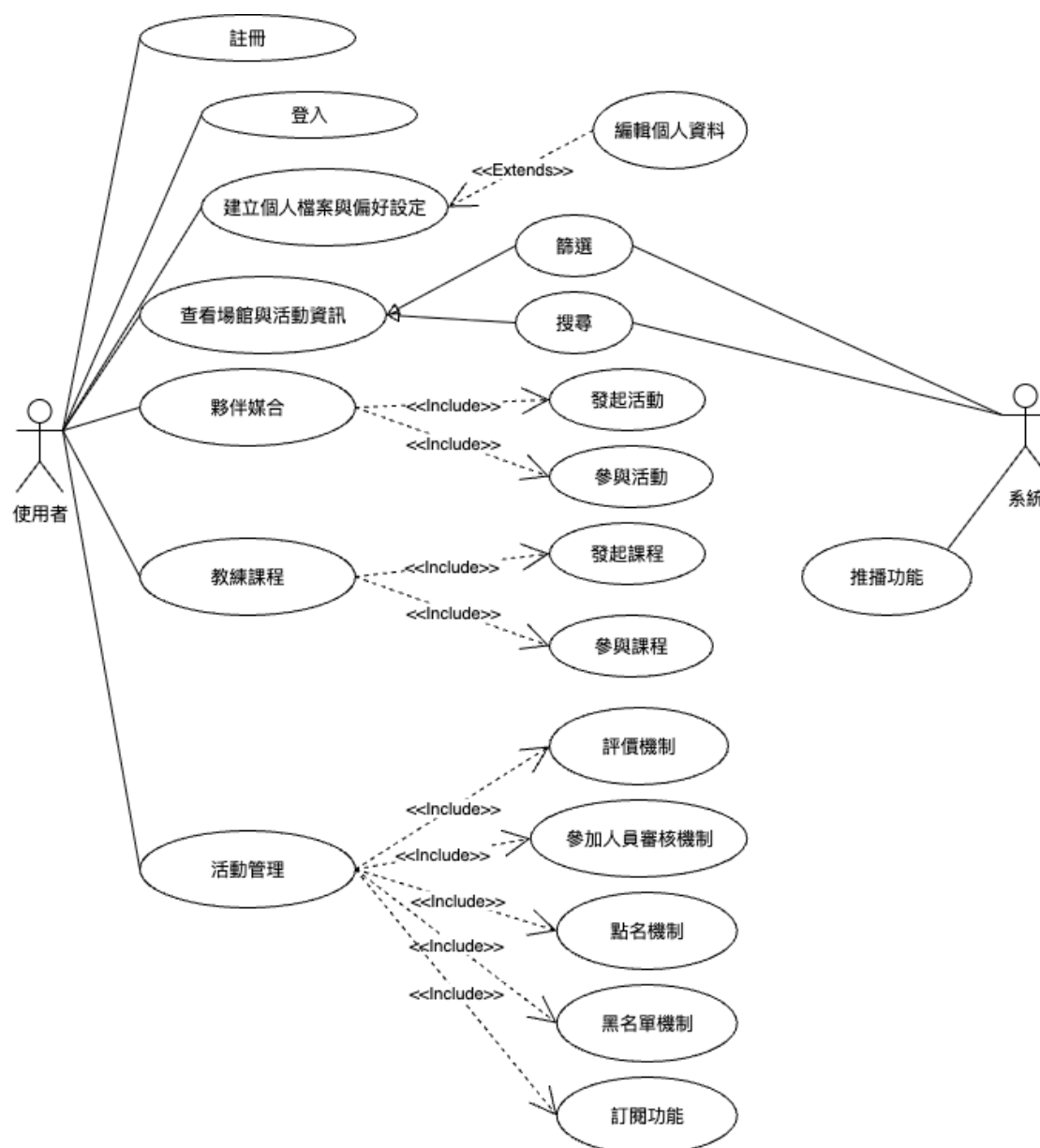
圖 5-2-1 使用個案圖
